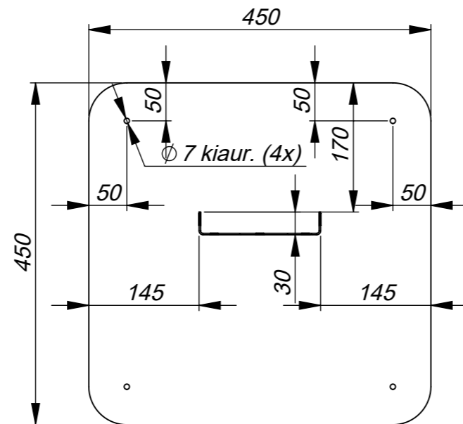
A-A 1:7
