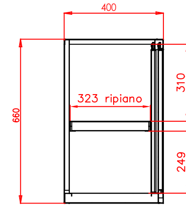
SEZIONE A-A
